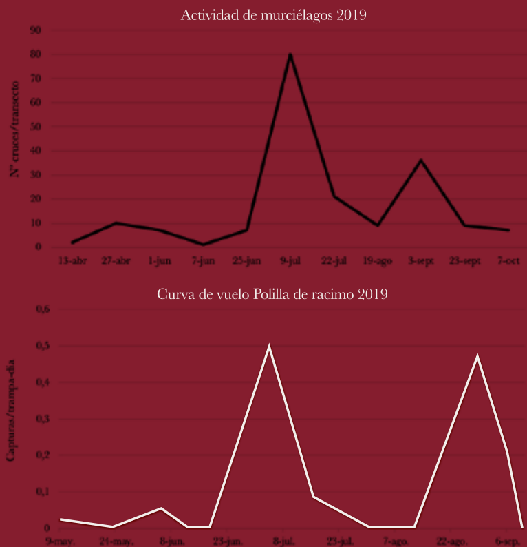
Figura 3: Evolución de la actividad de los murciélagos en función del tiempo y curva de vuelo de la polilla del racimo en Fontanars dels Alfòrns en 2019.
